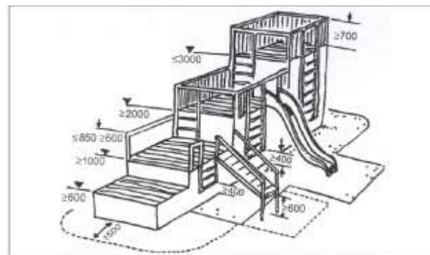
Hauteur de chute libre d'équipement d'aire de jeux pour des enfants de plus de 36 mois : schéma de synthèse.
